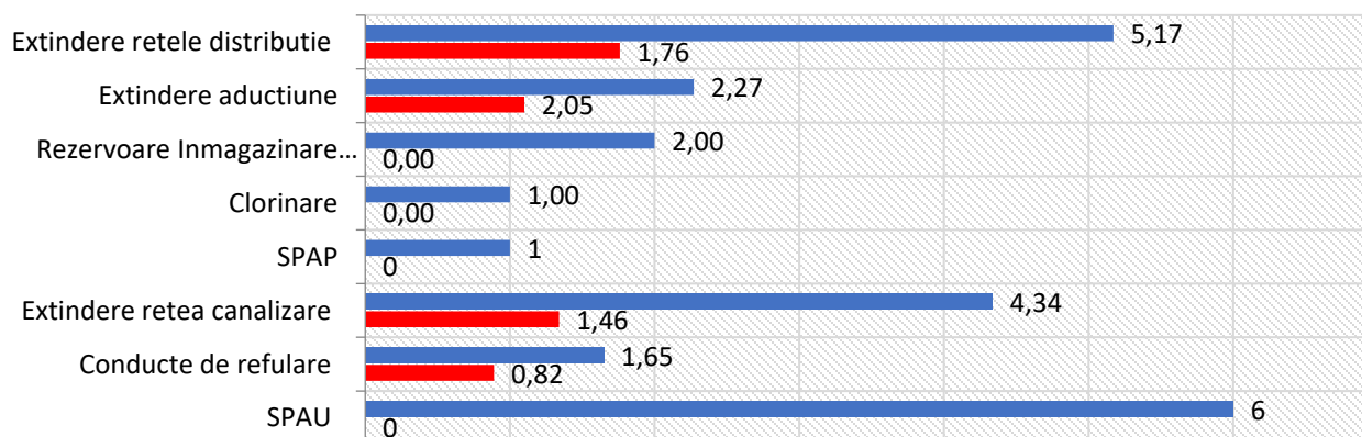
Stadiul realizării indicatorilor apă/canal - Moșoaia
